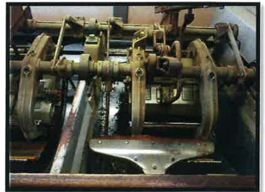
5 精揉機
